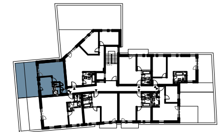
s ch é m a p ô d o r y s u 6 . N P / s c h e m e o f t h e s i x t h f l o o r
